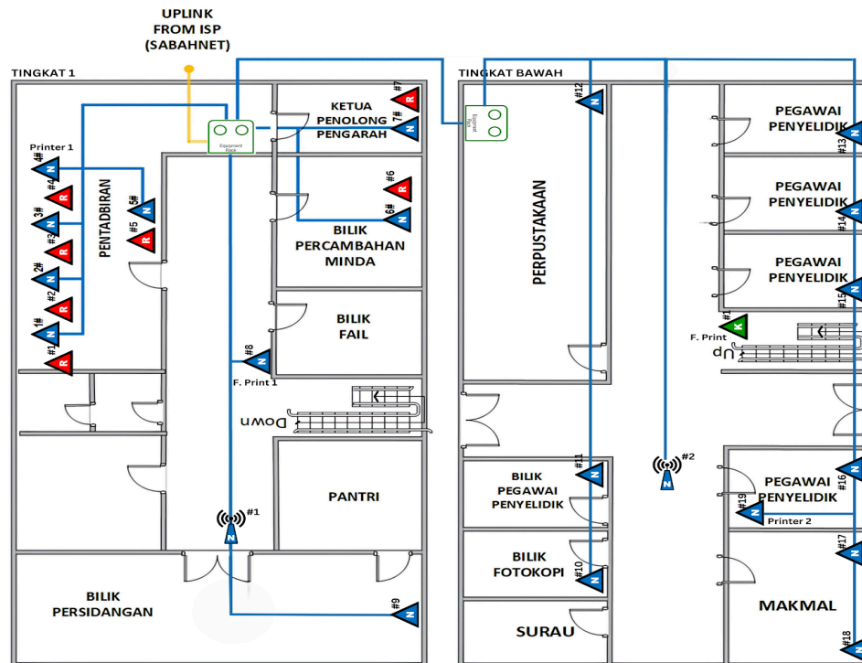
PELAN LANTAI CADANGAN BANGUNAN UTAMA PUSAT PENYELIDIKAN PERTANIAN BUKIT QUOIN, TAWAU
