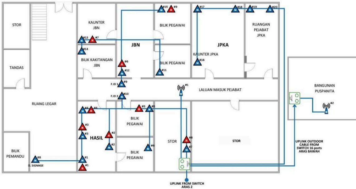
PELAN LANTAI CADANGAN PEJABAT DAERAH LAHAD DATU - ARAS BAWAH
